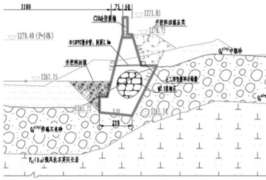
图 2-1 浆砌石衡重式防洪墙典型断面图
