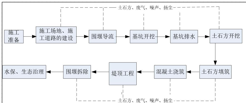
图 2-4 堤防施工工艺图
