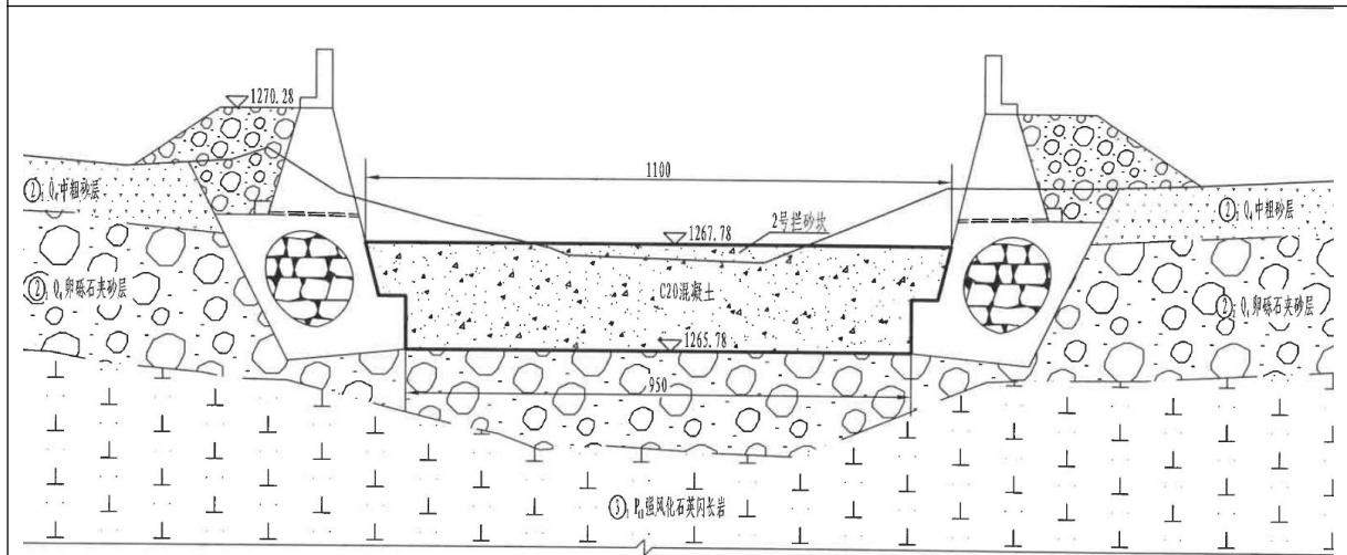
图 2-7 3号拦沙坝剖面图
