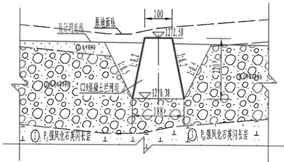
图 2-5 2 号拦沙坝剖面图
