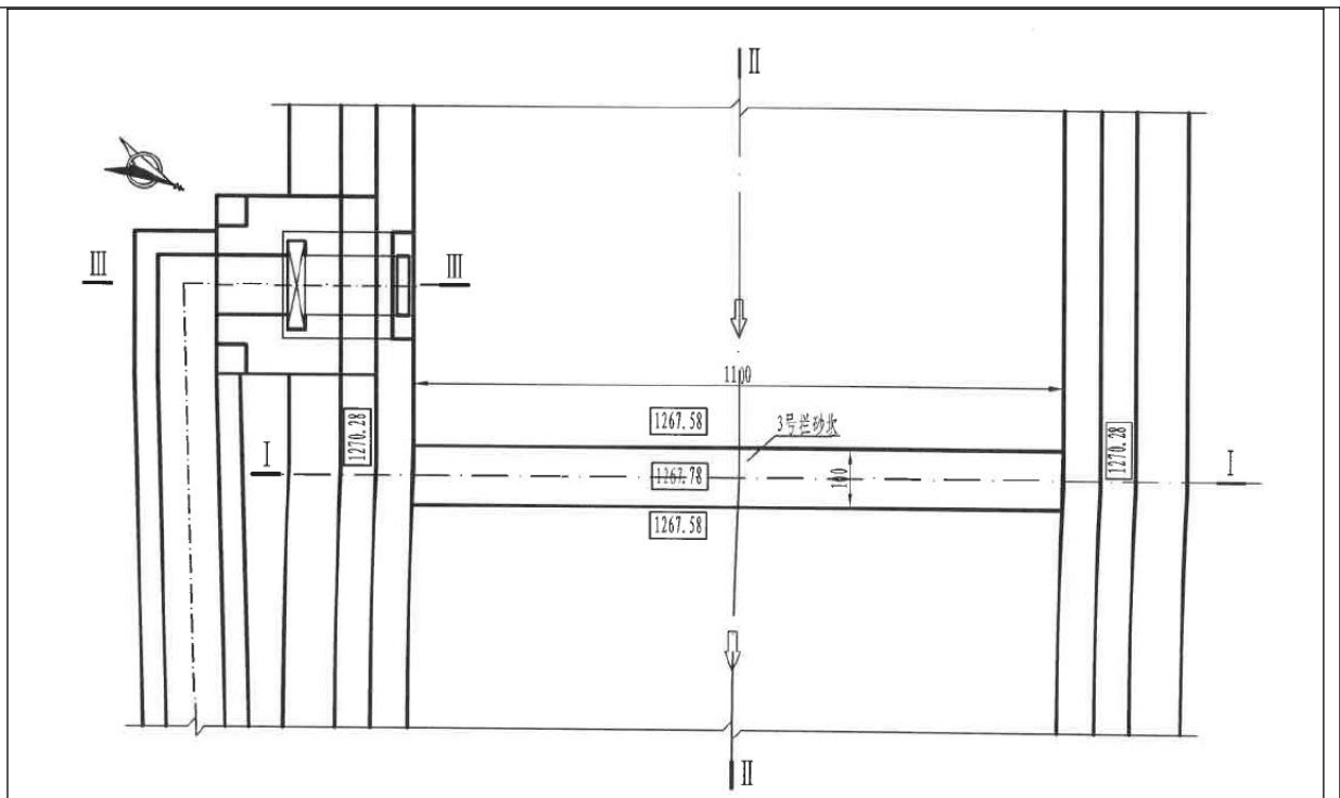
图 2-6 3号拦沙坝平面图
