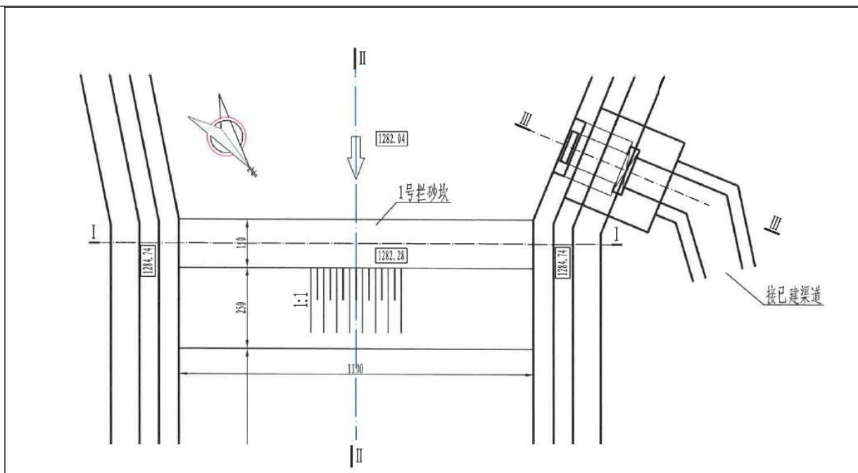
图 2-2 1 号拦砂坝平面图
