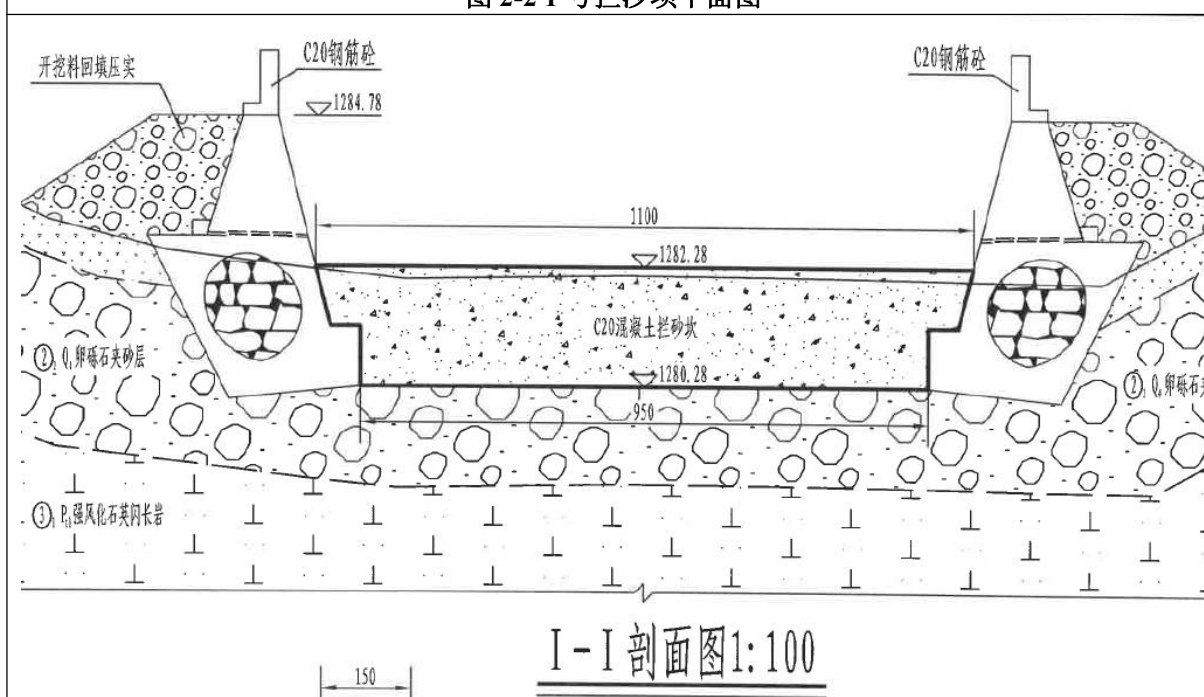
图 2-3 1 号拦砂坝剖面图
