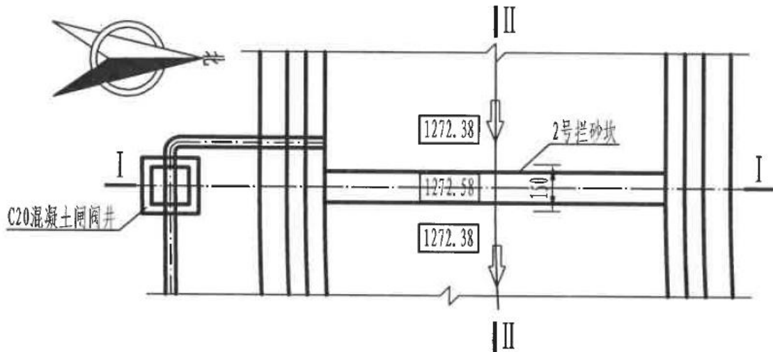
图 2-4 2 号拦沙坝平面图
