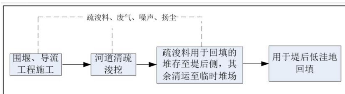
图 2-5 疏浚工艺流程及产污环节图
